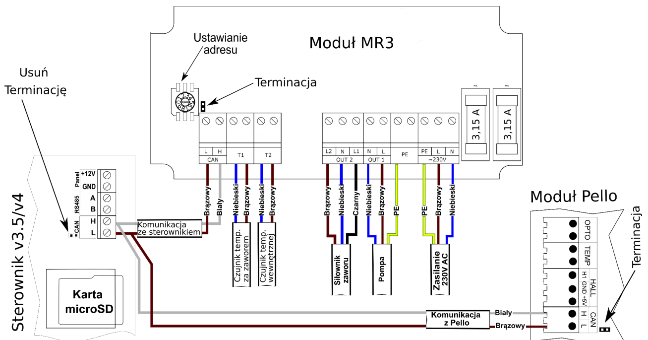
Ilustracja 14: Schemat podłączenia modułu rozszerzeń MR3 do sterownika v4.
