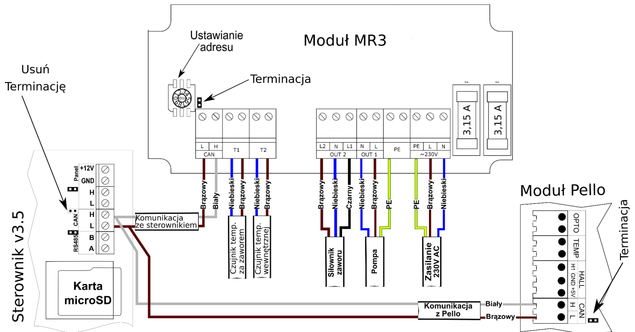
Ilustracja 13: Schemat podłączenia modułu rozszerzeń MR3 w sterowniku v3.5.
